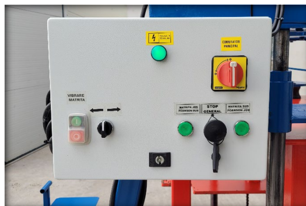
Accionare electrică, fără efort fizic, a matricei
