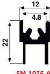
SM 1076 A 0,292 kg/m
