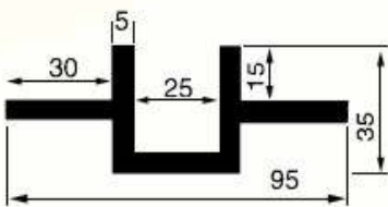
SB 5039 2,100 kg/m
