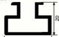
SM 1044 0,360 kg/m
