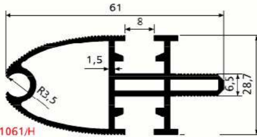
SM 1061/H 1.004 kg/m
