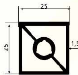
SK 706 0,585 kg/m
