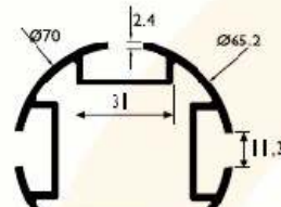
SB 5016 2,237 kg/m
