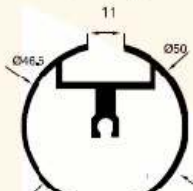
SM 5014 1,103 kg/m
