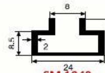
SM 1040 0,210 kg/m
