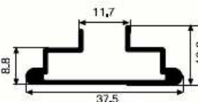
SM 1039 0,235 kg/m
