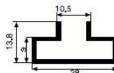
SM 1038 0,220 kg/m
