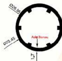
SM 5023 0,413 kg/m
