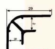
SM 1014 K 0,255 kg/m
