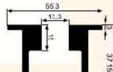
SM 1047 0,356 kg/m
