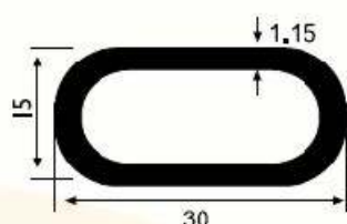
SM 1063 0,235 kg/m
