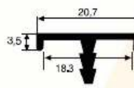
SM 1011 T 0,143 kg/m
