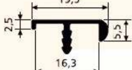
SM 1008/D 0,119 kg/m
