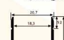
SM 1008 SJ 0,088 kg/m
