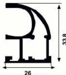
SM 1073 A 0,495 kg/m
