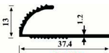
ST 204 0.180 kg/m
