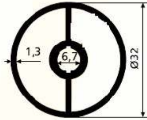
SK 5014/C 0.578 kg/m
