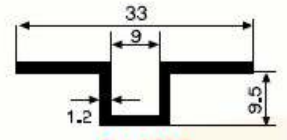
SM 1019 0,200 kg/m
