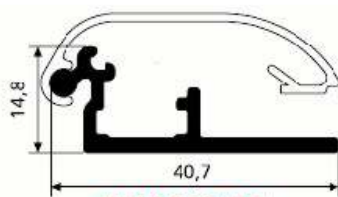
SM 1067/RM 0,363 kg/m
