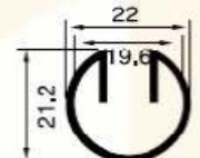
SB 5033 0.240 kg/m
