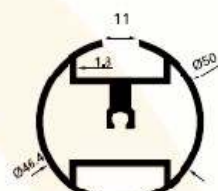
SM 5015 1,230 kg/m
