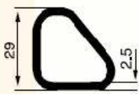
SB 5030 0,590 kg/m
