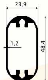
SM 1059 D 0,695 kg/m
