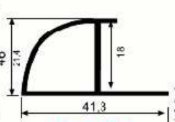
SM 1052 B 0,320 kg/m
