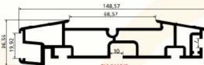
SM 5112/C 2,965 kg/m
