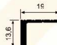
SM 1089 0.354 kg/m
