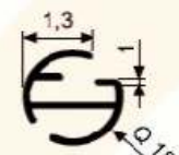
SB 5028 0.185 kg/m
