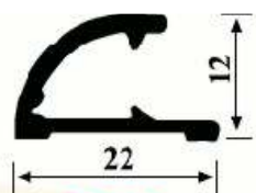
ST 203 0.170 kg/m
