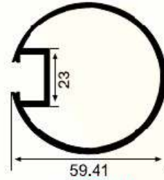
SM 1060 0,155 kg/m
