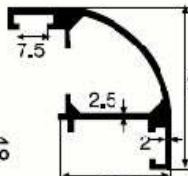
SM 1050 0,860 kg/m
