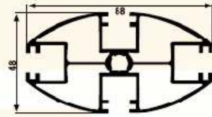
FS 4029 2,048 kg/m
