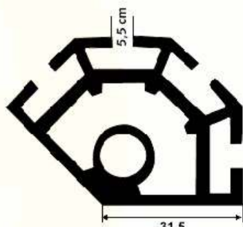
FS 4023 Kg/m 1.504
