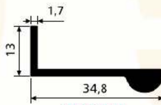
SM 1082/B 0.315 kg/m
