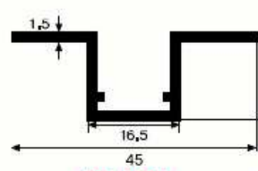
SM 1021 0,315 kg/m
