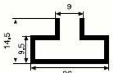
SM 1037 0,220 kg/m
