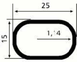
SM 1063 D 0,200 kg/m
