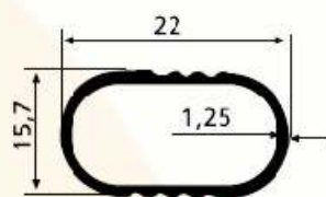
SM 1063 G 0,210 kg/m
