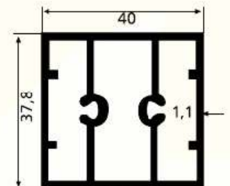
SK 707 0,760 kg/m
