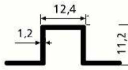
SM 1017 A 0,180 kg/m
