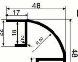
SM 1051 0,735 kg/m
