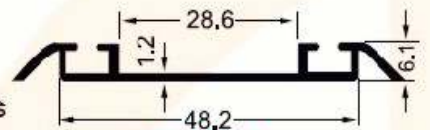
SM 1074 B 0,300 kg/m
