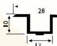
SM 1020 A 0,145 kg/m
