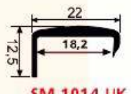
SM 1014 UK 0,190 kg/m
