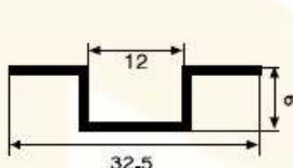
SM 1020 0,135 kg/m
