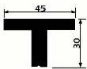
SM 6013 I 1,460 kg/m
