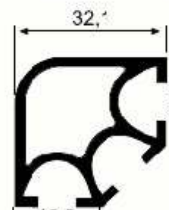
23 D 3 0,670 kg/m
