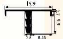
SM 1014 S 0,100 kg/m
