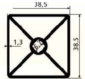
SK 709 1.019 kg/m
