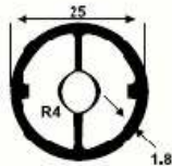
SM 1063 B 0,520 kg/m
