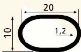
SM 1063 F 0,160 kg/m
