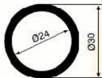
SM 5025 0,687 kg/m
