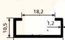
SM 1055/N 0,177 kg/m
