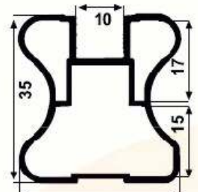
SM 1073 B 0,501 kg/m
