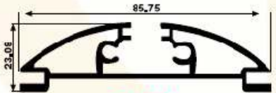
FS 4030 1,044 kg/m
