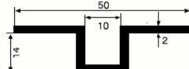
SM 1018 0,440 kg/m
