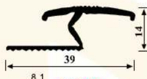
ST 206 0.240 kg/m
