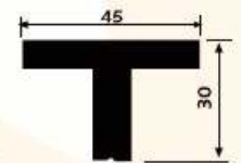
SM 6013 H 1,580 kg/m
