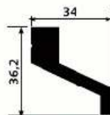
SM 6013 J 0,980 kg/m
