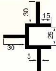
SB 5038 2,510 kg/m
