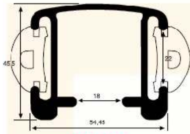
SM 7029 1,615 kg/m
