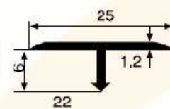
SM 1022 0,100 kg/m
