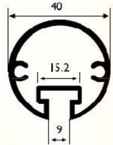
SM 1060 B 0,740 kg/m
