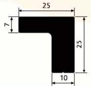
SM 6013 G 0,700 kg/m
