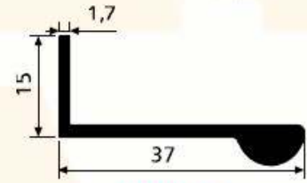
SM 1082/C 0.335 kg/m
