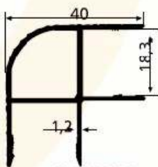
SM 1052 E 0,510 kg/m
