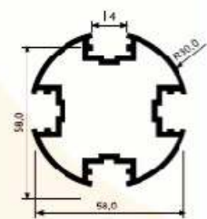
SB 5019 1,504 kg/m
