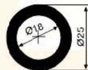
SM 5026 0,638 kg/m
