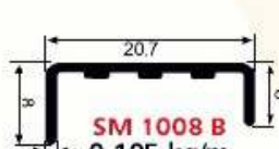
SM 1008 B 0,105 kg/m
