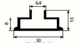
SM 1041 0,185 kg/m
