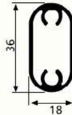
SM 1059 C 0,510 kg/m
