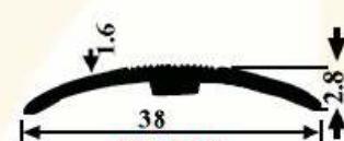
ST 217 0.180 kg/m
