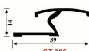
ST 205 0.270 kg/m
