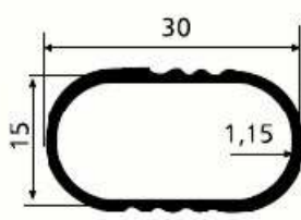
SM 1063 A 0,235 kg/m
