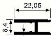
SM 1086 0.152 kg/m
