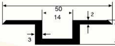
SM 1017 0,470 kg/m
