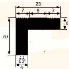
SM 6013 M 0,594 kg/m
