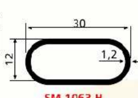
SM 1063 H 0,230 kg/m
