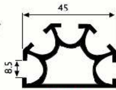
21 D 5 0,900 kg/m
