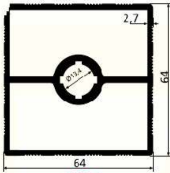
SK 710 0.664 kg/m
