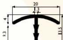
SM 1023 A 0,125 kg/m
