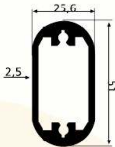
SM 1059 1,130 kg/m
