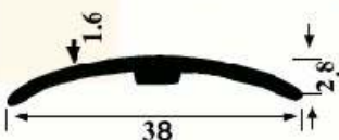
ST 216 0.290 kg/m
