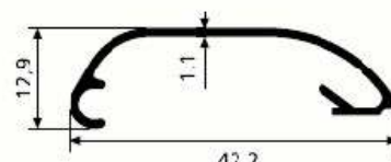
SM 1067/R 0,218 kg/m
