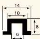
SM 1097 0.140 kg/m
