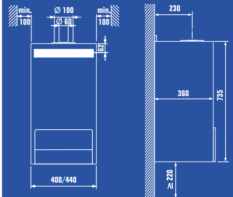
Logamax U052
